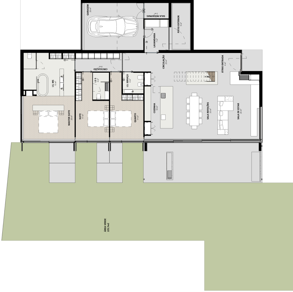
1 | 1:100 PLANTA PISO 0 (FRAÇÃO D) | ABC - 250m 2 | AU - 227m 2
